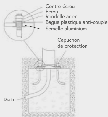
Fig. 1 : Mât aluminium
