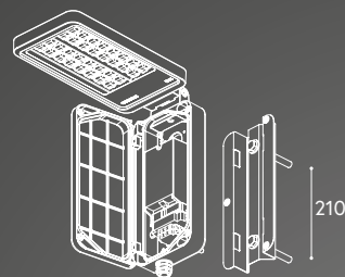
Kit boulons traversants (pour perçages mâts béton normalisés et mâts bois cylindroconiques)
