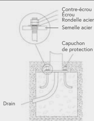
Fig. 2 : Mât acier
